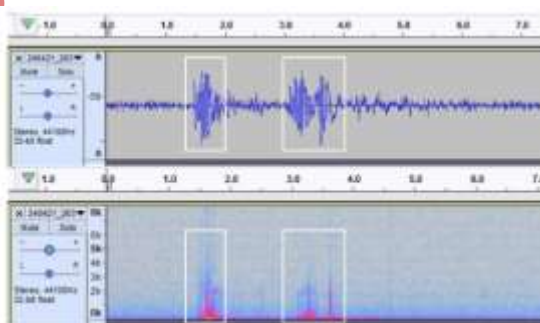
شکل ۴. شماتیک تحلیل داده‌های صوتی در نرم‌افزار Audacity. (الف) نمای شکل موج؛ (ب) نمای طیف‌نگاره؛ (ج) انتخاب بازه موردنظر و (د) Spectrum/Frequency Analysis دامنه را برحسب بسامد نمایش می‌دهد.
